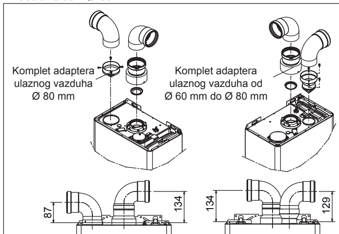
Dvostruke cevi Ø 80 mm
