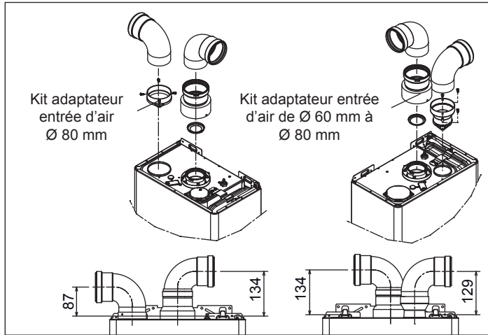
Longueur maximale tuyaux ø 80 mm - 25 KIS
