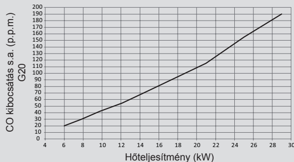
Kibocsátás - hőteljesítmény-görbe (MTN)
