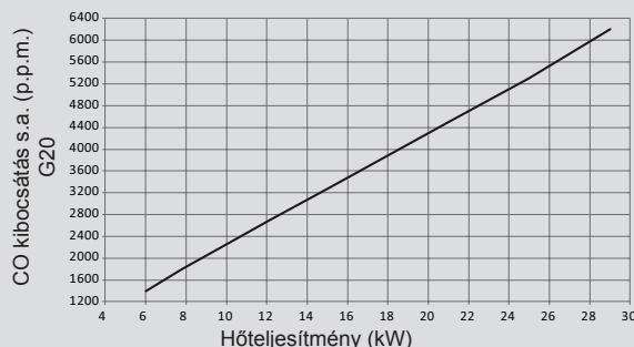
Hőteljesítmény-görbe – ventilátor fordulatszáma (MTN)
