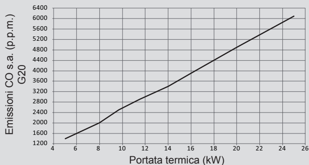
Curva portata termica - nr. giri ventilatore (MTN)
