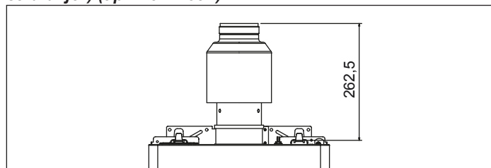
Cev za odvod dimnih gasova Ø 80 mm (instalacija „forsirano otvaranje“) (tip B23P-B53P)
