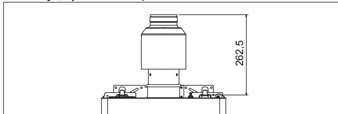
Vod za ispušt dimnih plinova Ø 80 mm ("prisilna otvorena" instalacija; tip B23P-B53P)
