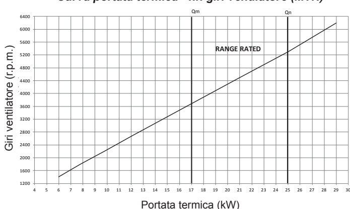
Curva portata termica - nr. giri ventilatore (MTN)
