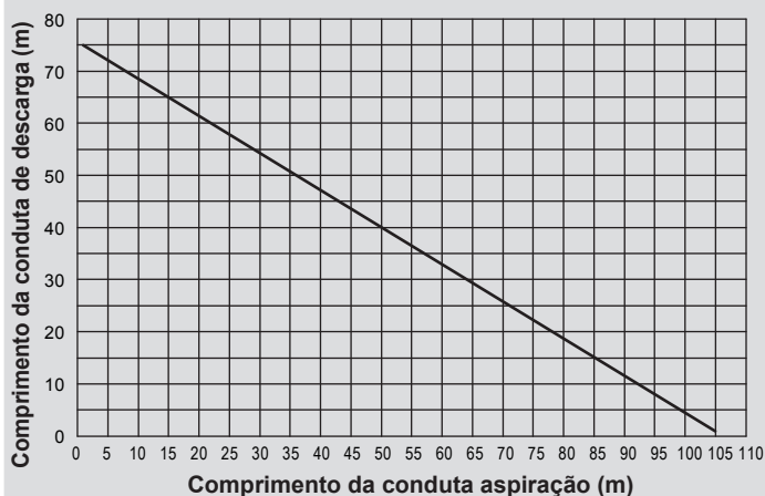
Comprimento máximo dos tubos Ø 80 mm - 29 KIS
