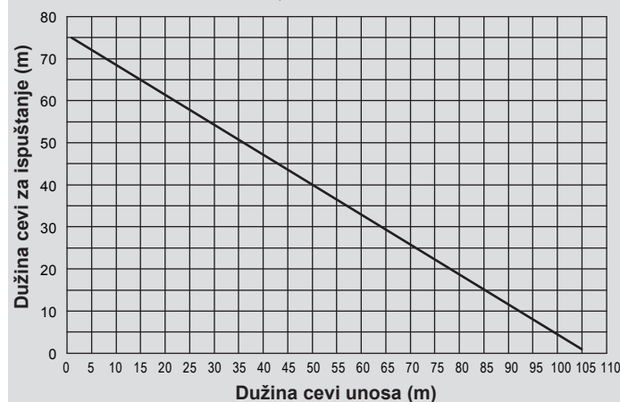
Maksimalna dužina cevi Ø 80 mm - 25 KIS
