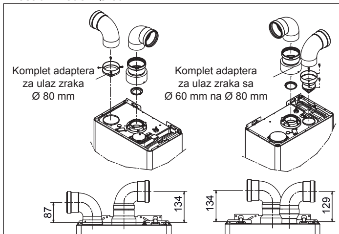
Dvostruki vodovi Ø 80 mm
