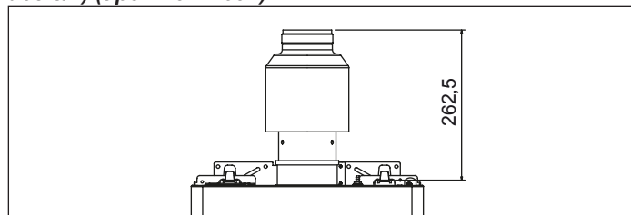
Conduta de descarga de fumos Ø 80 mm (instalação "forçada aberta") (tipo B23P-B53P)
