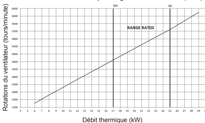
Courbe de débit calorifique - régime du ventilateur (MTN)
