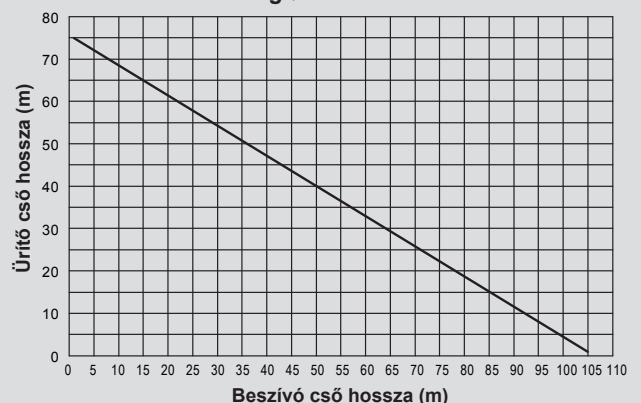
Maximális csőhosszúság Ø 80 mm - 25 KIS
