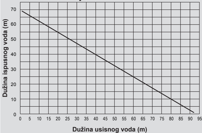
Maksimalna dužina cijevi Ø 80 mm - 29 KIS
