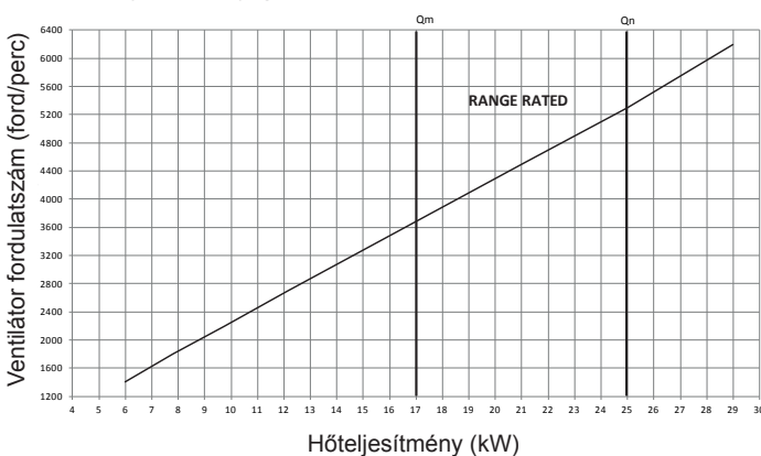
Hőteljesítmény-görbe – ventilátor fordulatszáma (MTN)
