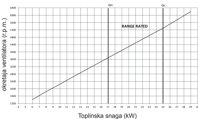
Krivulja toplinske snage - br. okretaja ventilatora (MTN)
