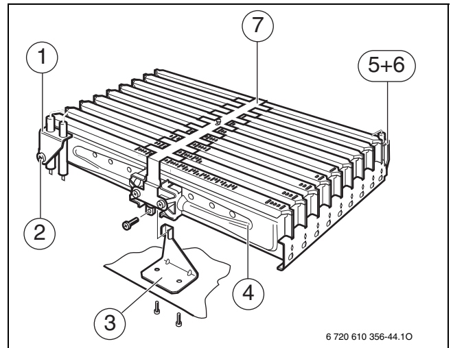
Fig. 34 Blocco bruciatore
