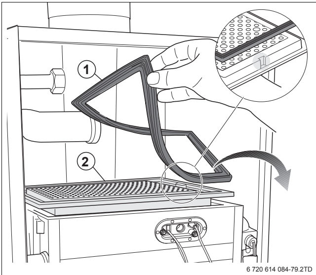
Fig. 64 Rimuovere il bruciatore e la relativa guarnizione
