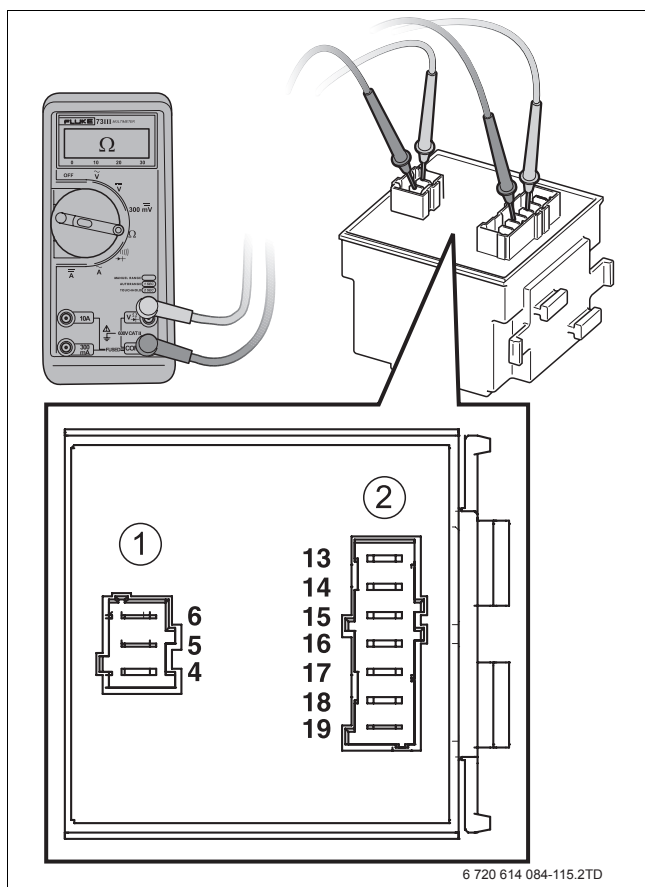
Fig. 81 Controllo trasformatore
