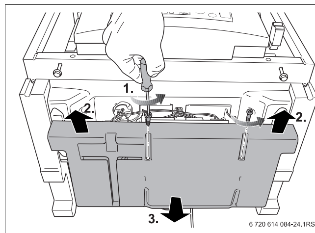
Fig. 19 Rimuovere la copertura della morsettiere
