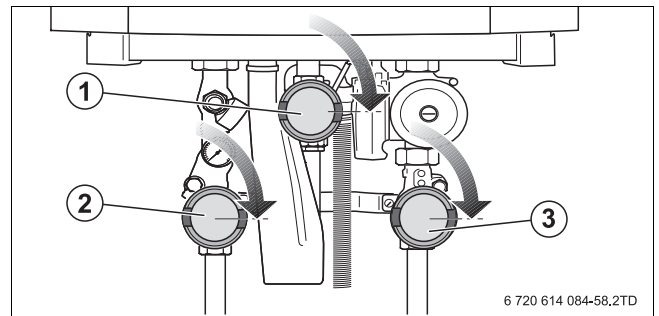
Fig. 53 Chiudere i rubinetti
