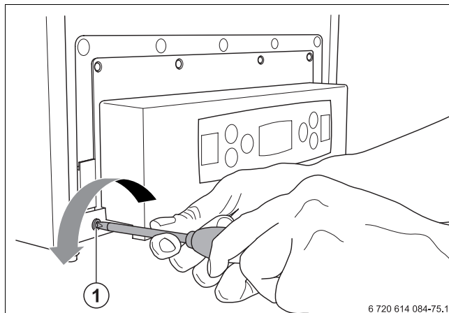
Fig. 70 Smontare l'unità di servizio
