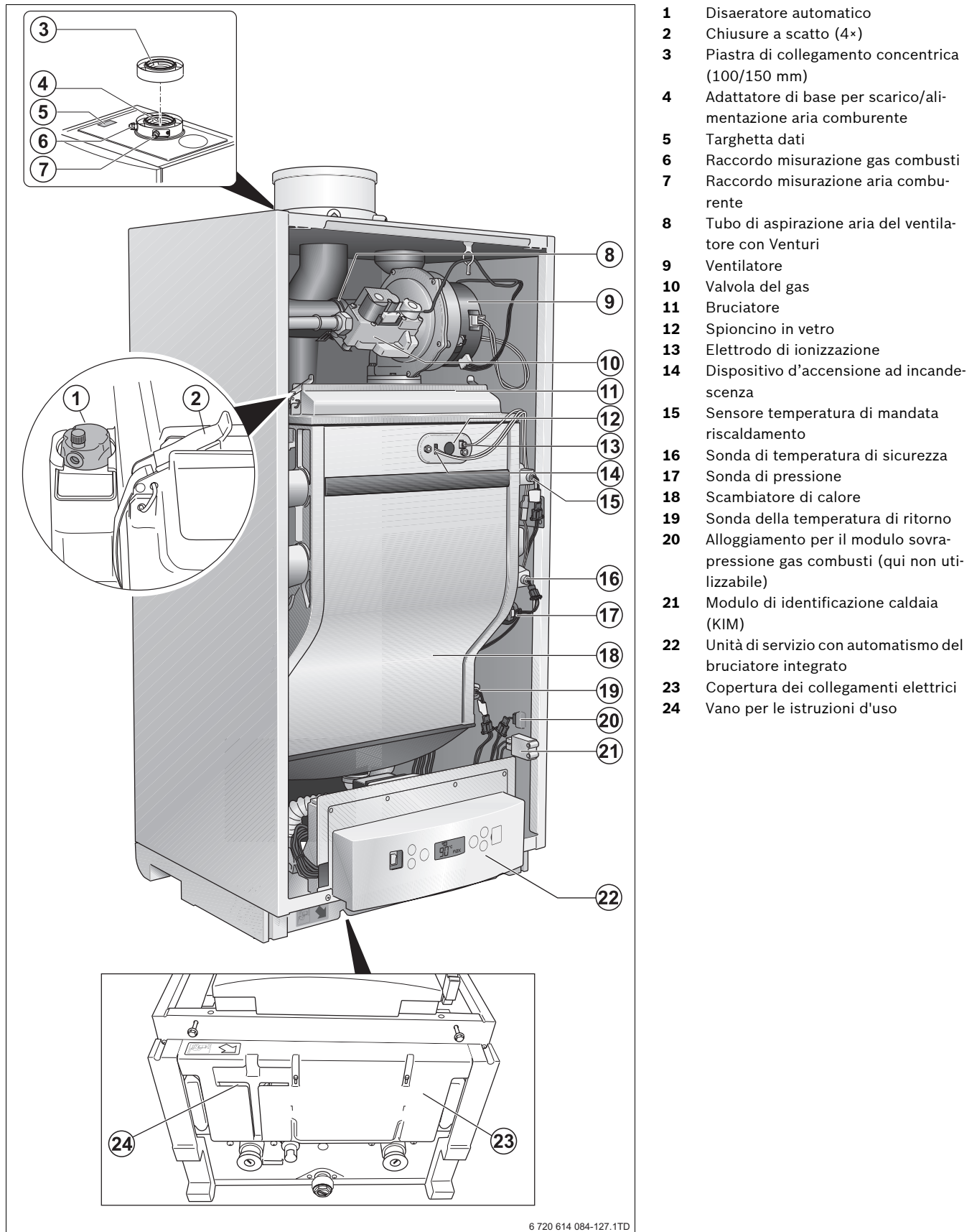
Fig. 1 Panoramica prodotto CerapurMaxx
