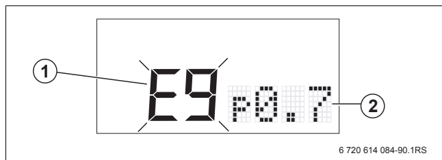
Fig. 74 Indicazione delle anomalie sul display
