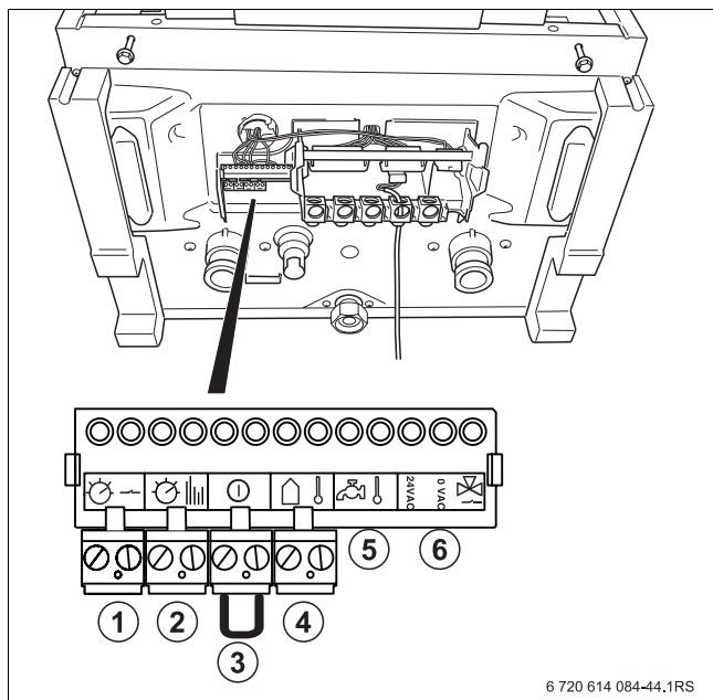
Fig. 20 Morsettiere bassa tensione
