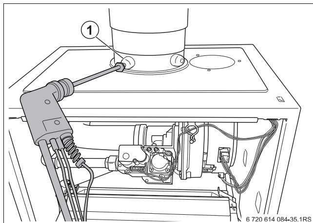
Fig. 45 Punto di misurazione per i gas di scarico
