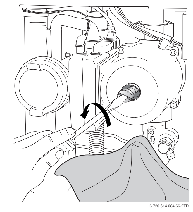
Fig. 36 Disaerare la pompa
