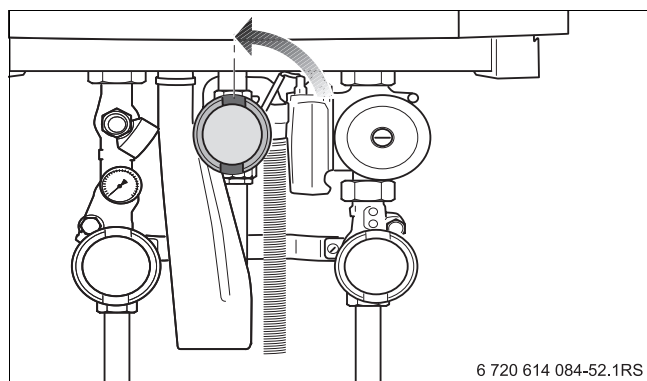
Fig. 37 Aprire il rubinetto del gas (qui con il gruppo di collegamento)
